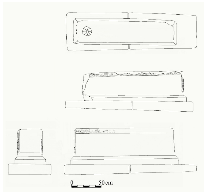
Рис. 9. Мраморное надгробие у входа в мавзолей Аль-Ходжа-ата. Чертеж [Fig. 9. Marble tombstone at the entrance to the Al-Khoja-Ata Mausoleum. Drawing]
