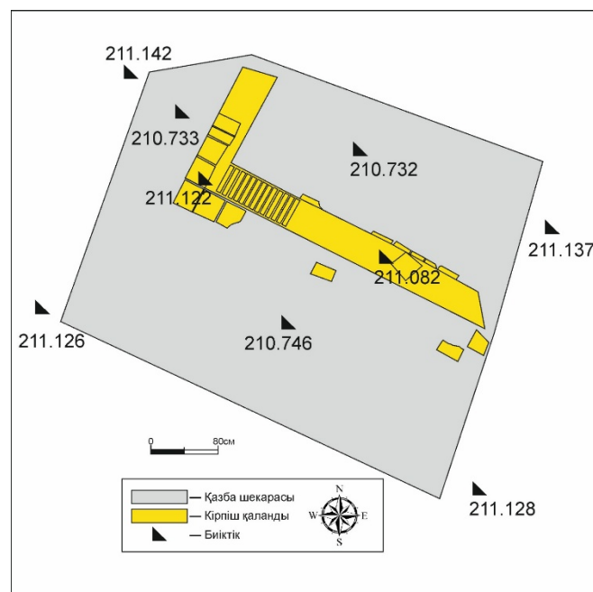
Рис. 5. План раскопанной стены. Мавзолей Али-Ходжа-Ата [Fig. 5. Plan of the excavated wall. Ali-Khoja-Ata Mausoleum]
